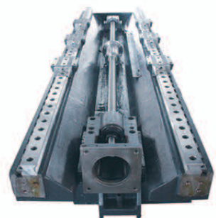
鞍座
